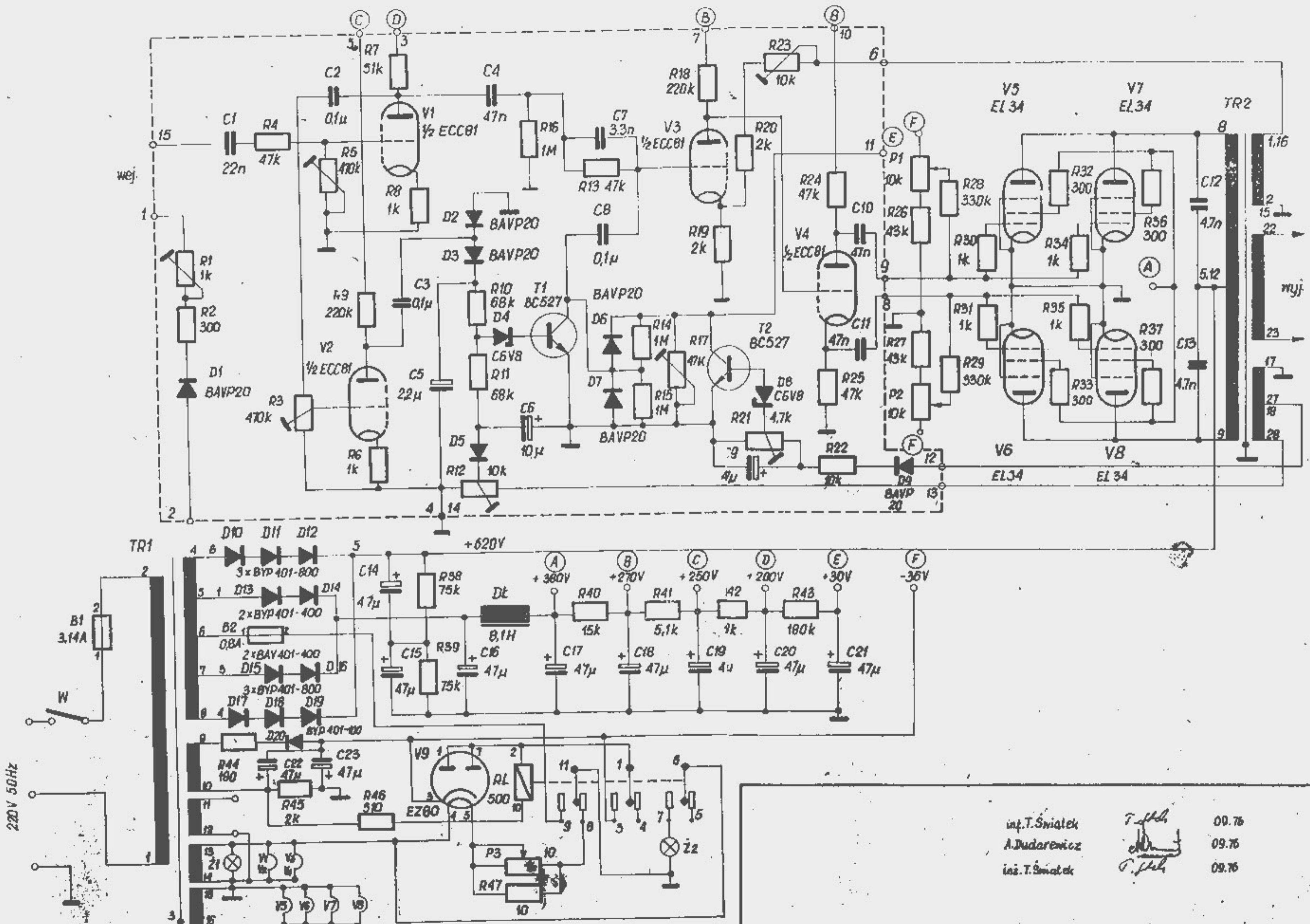
Schemat ideowy wzmacniacza BIS-101 45-0001-01
